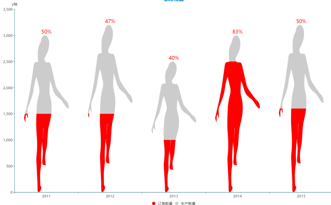
象形柱图
